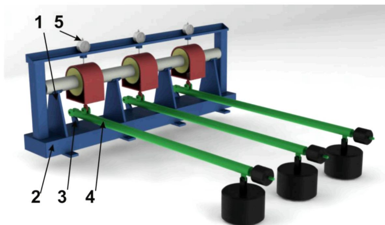
Рисунок Б3 – Установка для испытаний образцов на радиальную ползучесть
